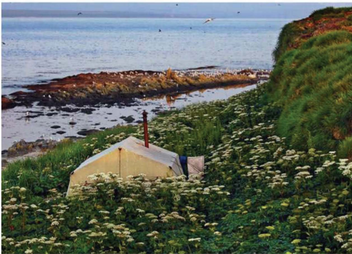
Лагерь исследователей на острове Топорков: с мая по август температура редко поднимается выше плюс десяти; в воздухе стоит полутуман, полудождь. Несмотря на то что есть печка, в палатке все равно часто бывает сыро
