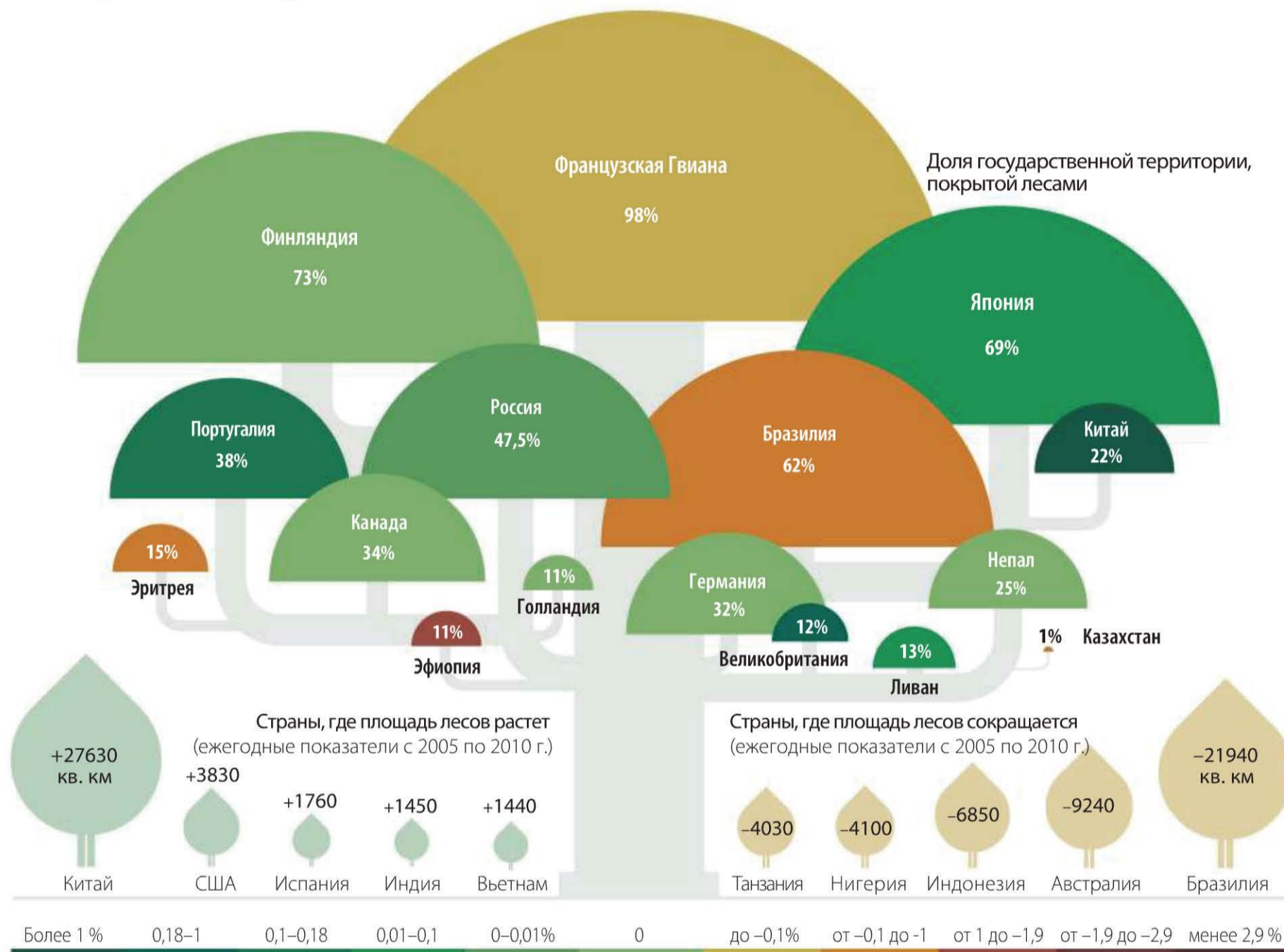
Ежегодное изменение процентной доли лесных площадей в период 2005—2010 годов
