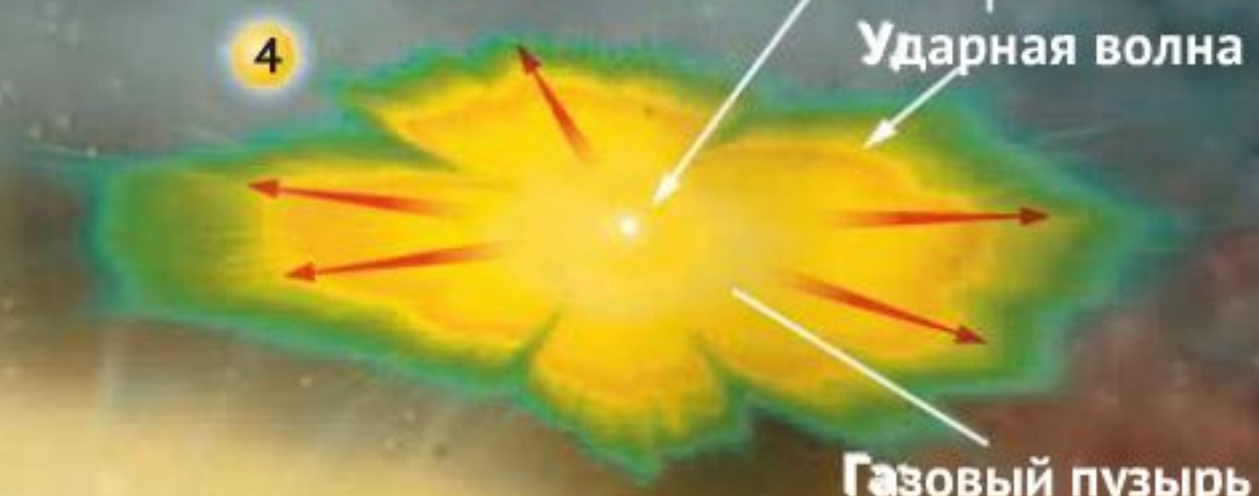
Нейтронная звезда
