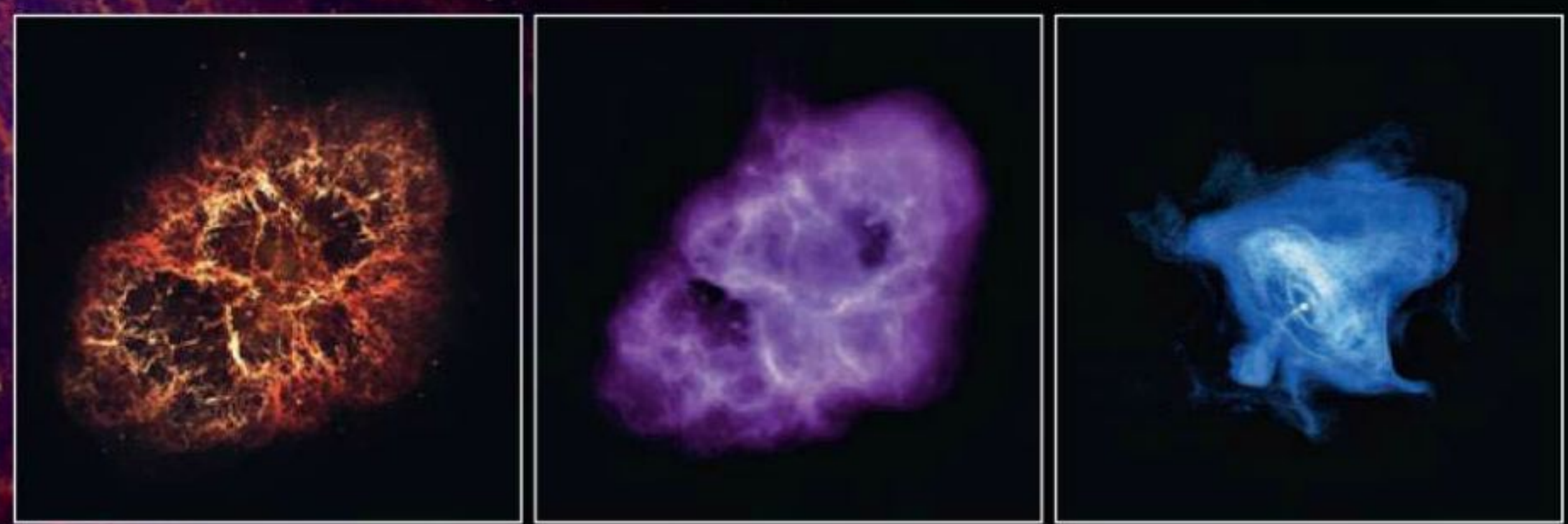
Гигантская Крабовидная туманность в созвездии Тельца образовалась в результате взрыва сверхновой. Ее вспышка наблюдалась в 1054 году даже днем. Это газовое облако, расширяющееся со скоростью 1500 километров в секунду, светится в двух диапазонах: оптическом (фото слева) и инфракрасном (в середине). В его центре находится нейтронная звезда — сжатое ядро первоначального светила. Оно испускает энергонасыщенное рентгеновское излучение (справа)
